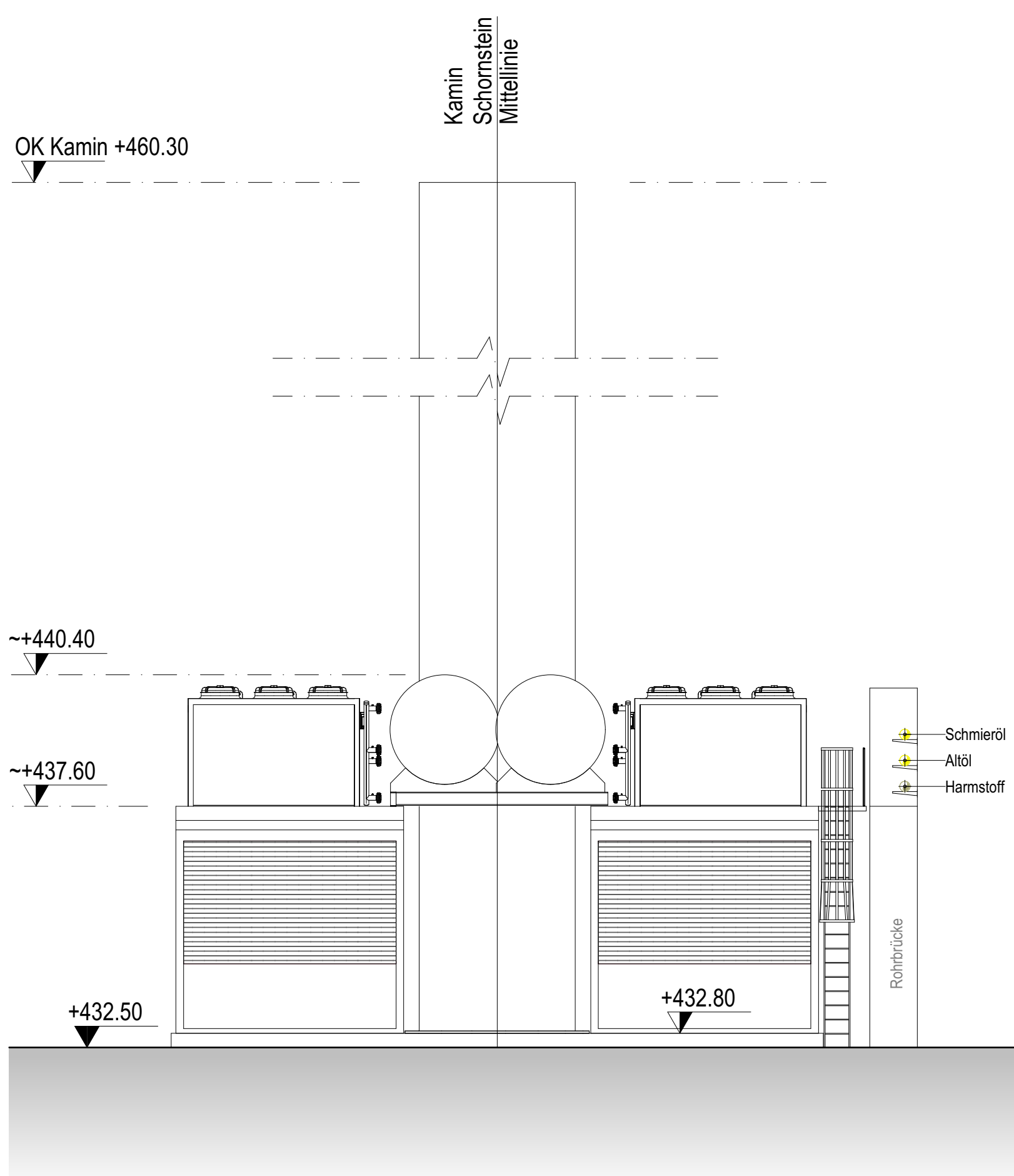
Ansicht Ost und West
