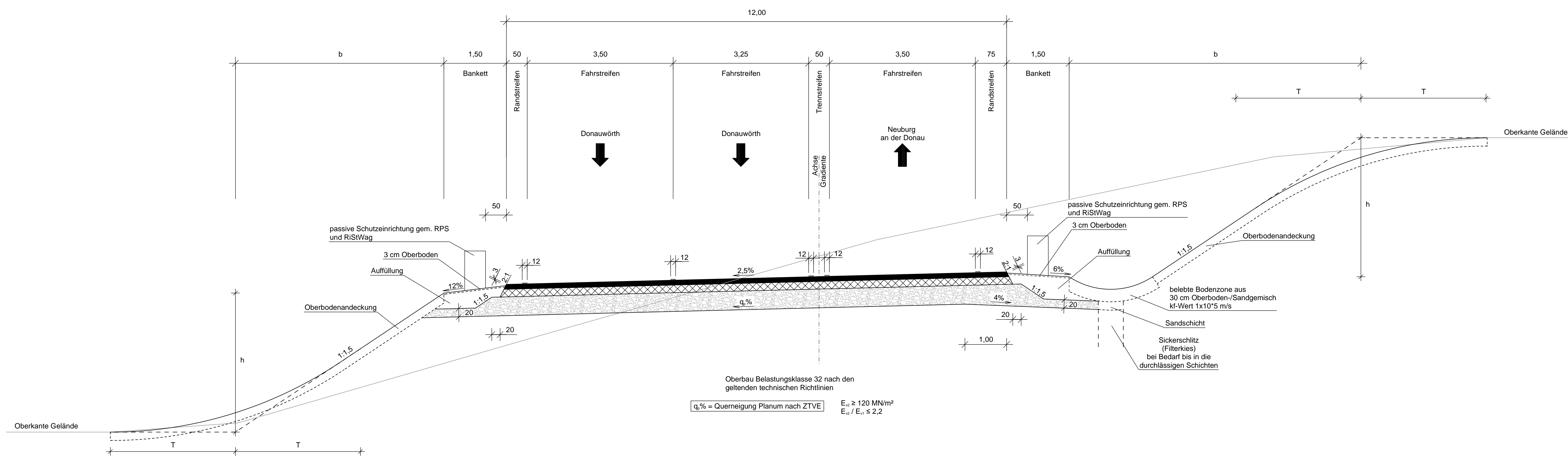
Regelquerschnitt B 16 (RQ 11.5+ mit ÜFS), M 1 : 50
