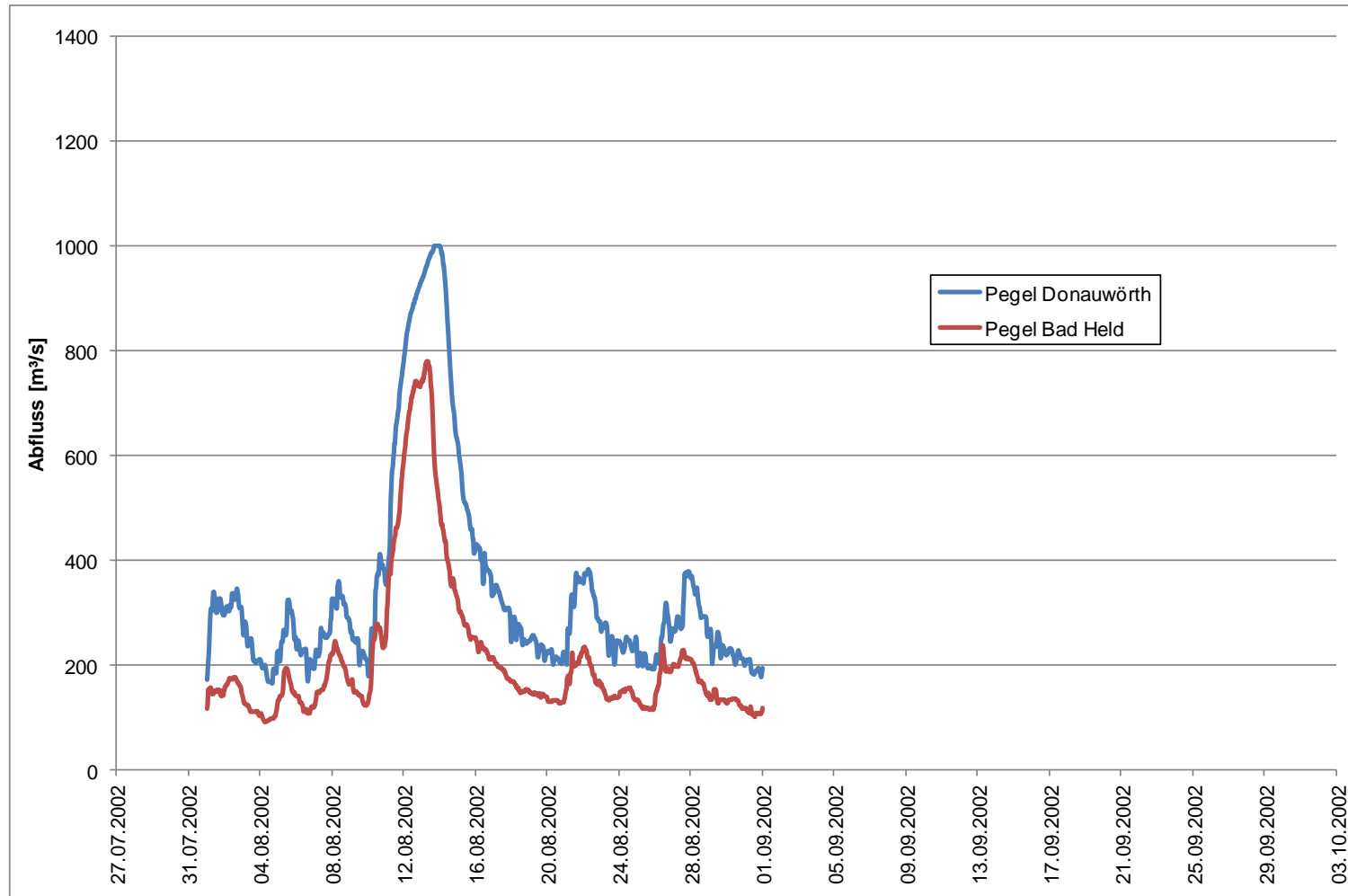
Anlage 3.1.5: Abflussganglinien Hochwasser August 2002, Pegel Bad Held und Donauwörth
