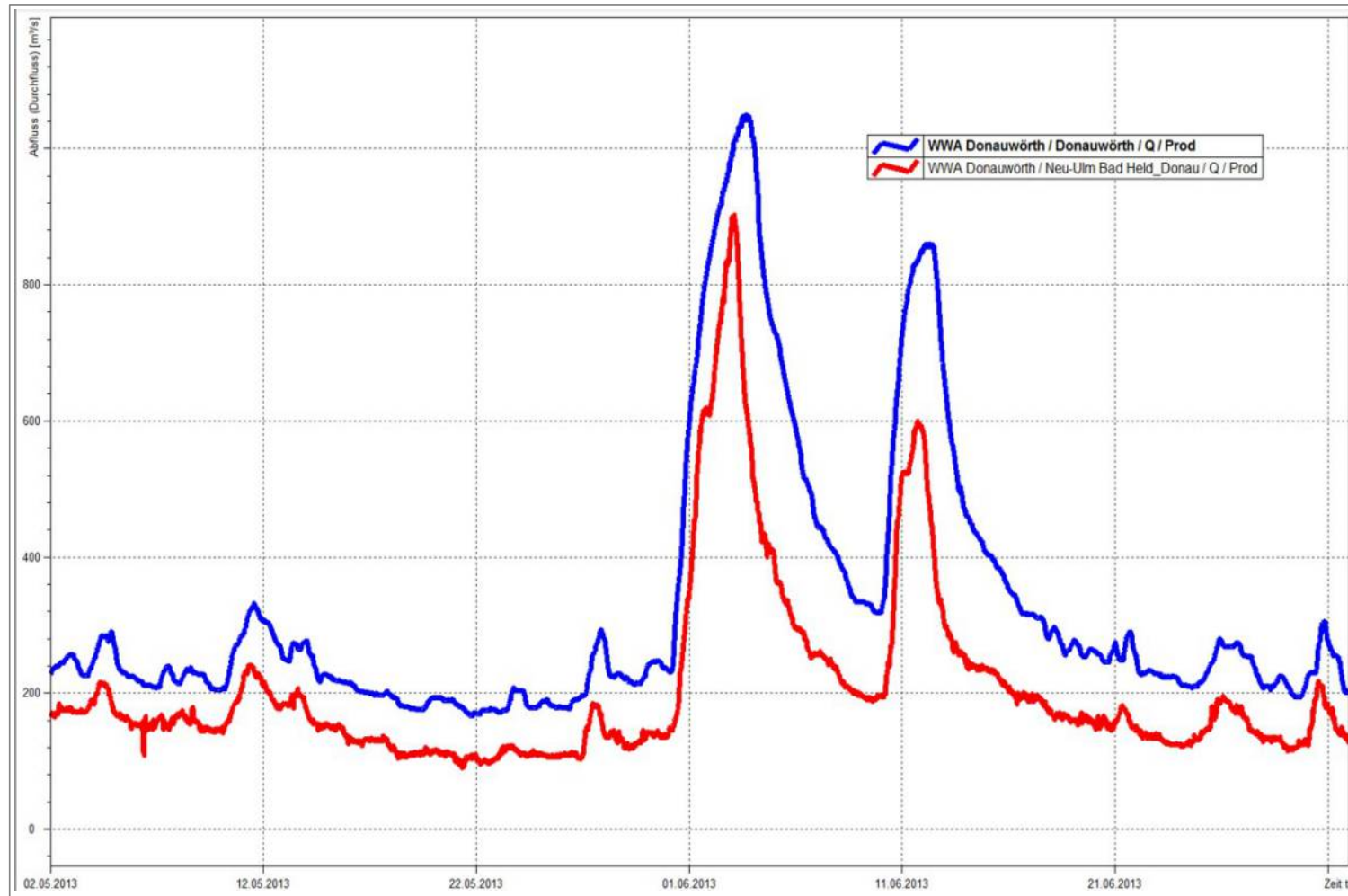
Anlage 3.1.7: Abflussganglinien Hochwasser Juni 2013, Pegel Bad Held und Donauwörth
