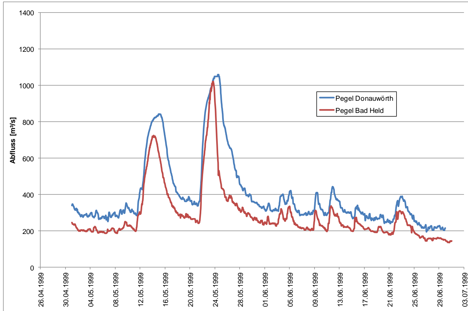
Anlage 3.1.4: Abflussganglinien Hochwasser Mai/Juni 1999, Pegel Bad Held und Donauwörth
