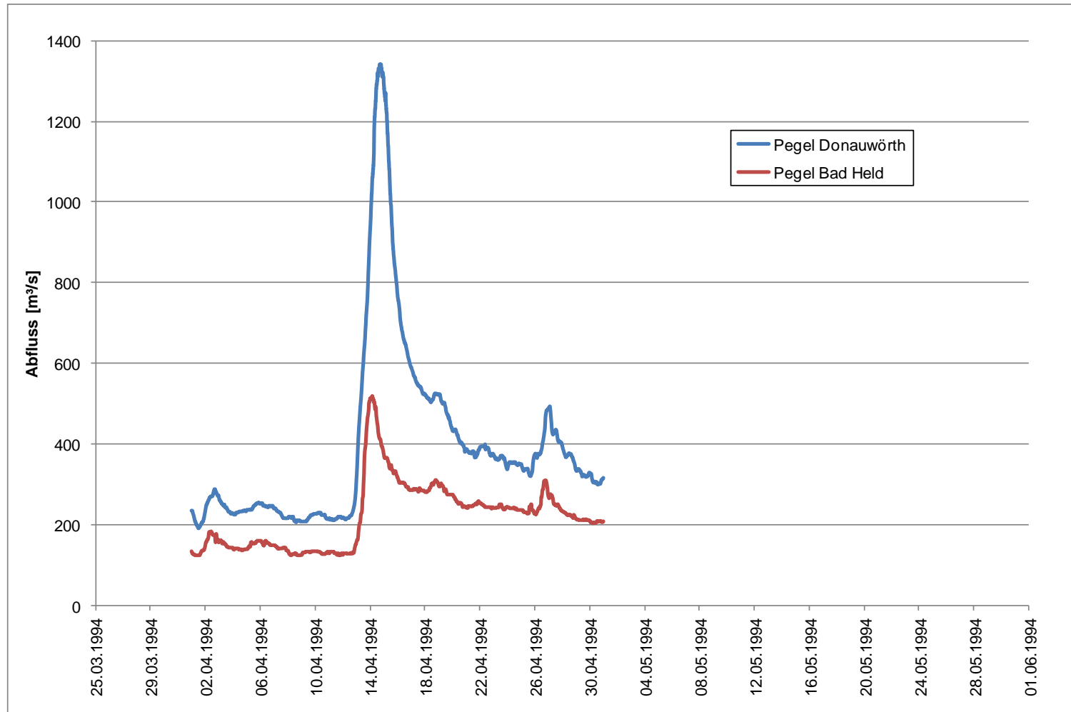
Anlage 3.1.3: Abflussganglinien Hochwasser April 1994, Pegel Bad Held und Donauwörth
