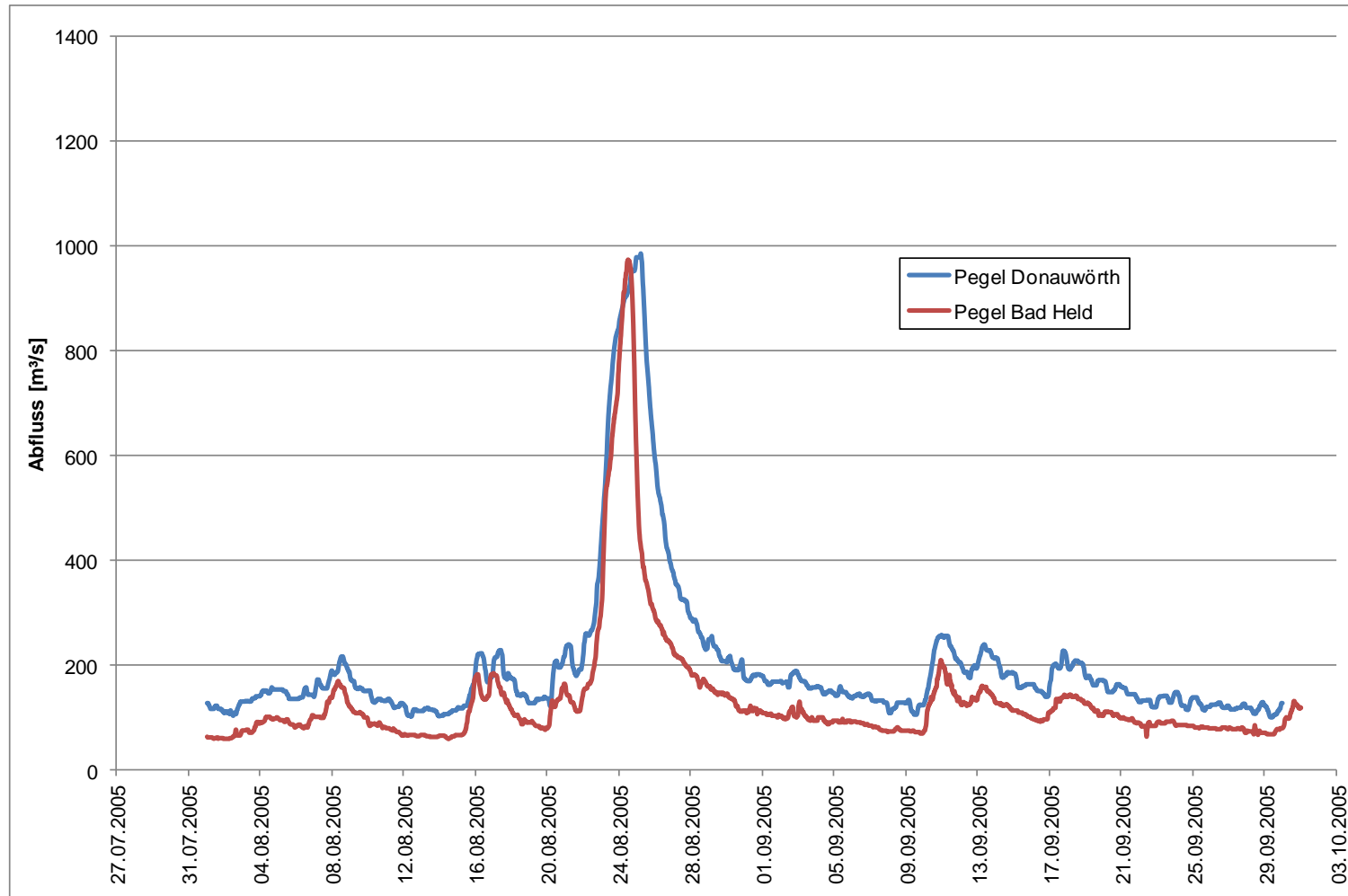
Anlage 3.1.6: Abflussganglinien Hochwasser August 2005, Pegel Bad Held und Donauwörth
