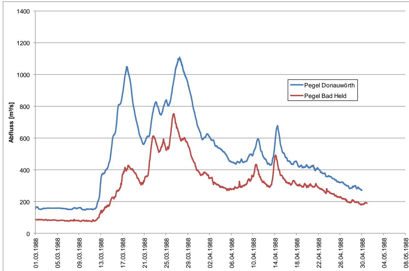
Anlage 3.1.1: Abflussganglinien Hochwasser März / April 1988, Pegel Bad Held und Donauwörth
