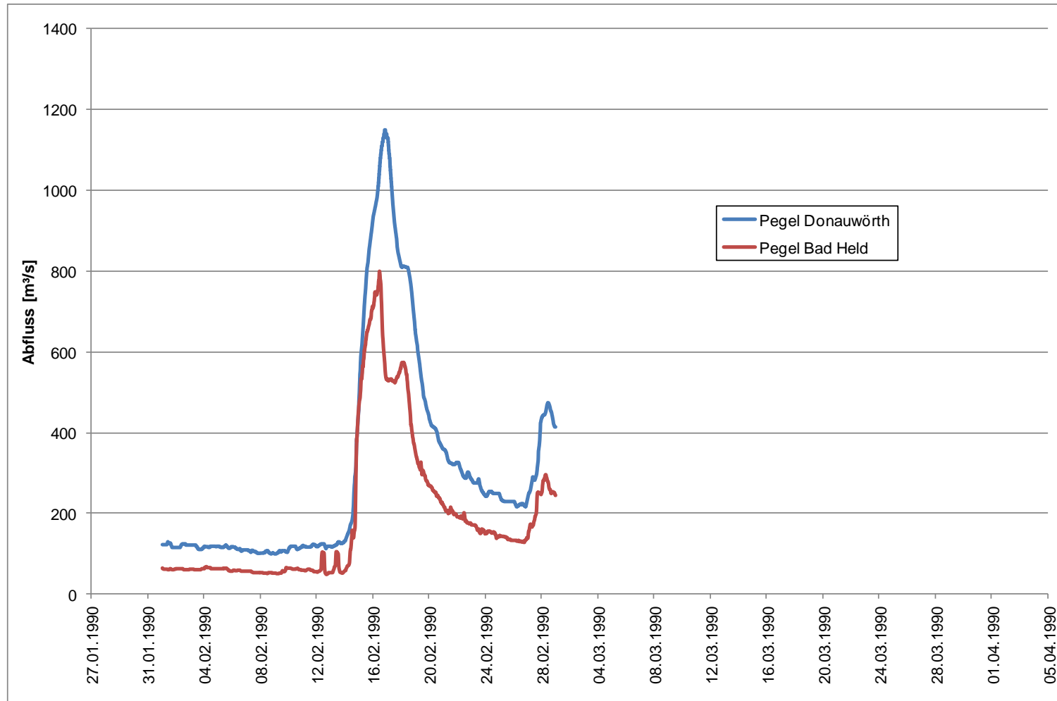
Anlage 3.1.2: Abflussganglinien Hochwasser Februar 1990, Pegel Bad Held und Donauwörth
